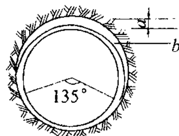
图 6.3.7 超挖示意图
