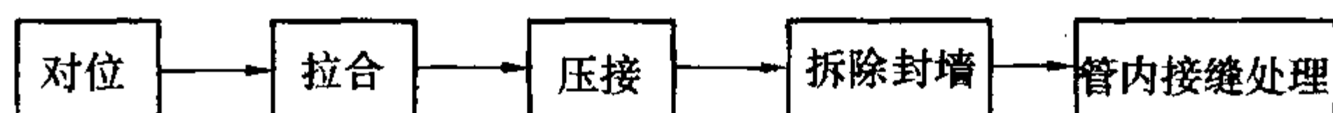
图 7.2.7 水力压接法主要施工程序
