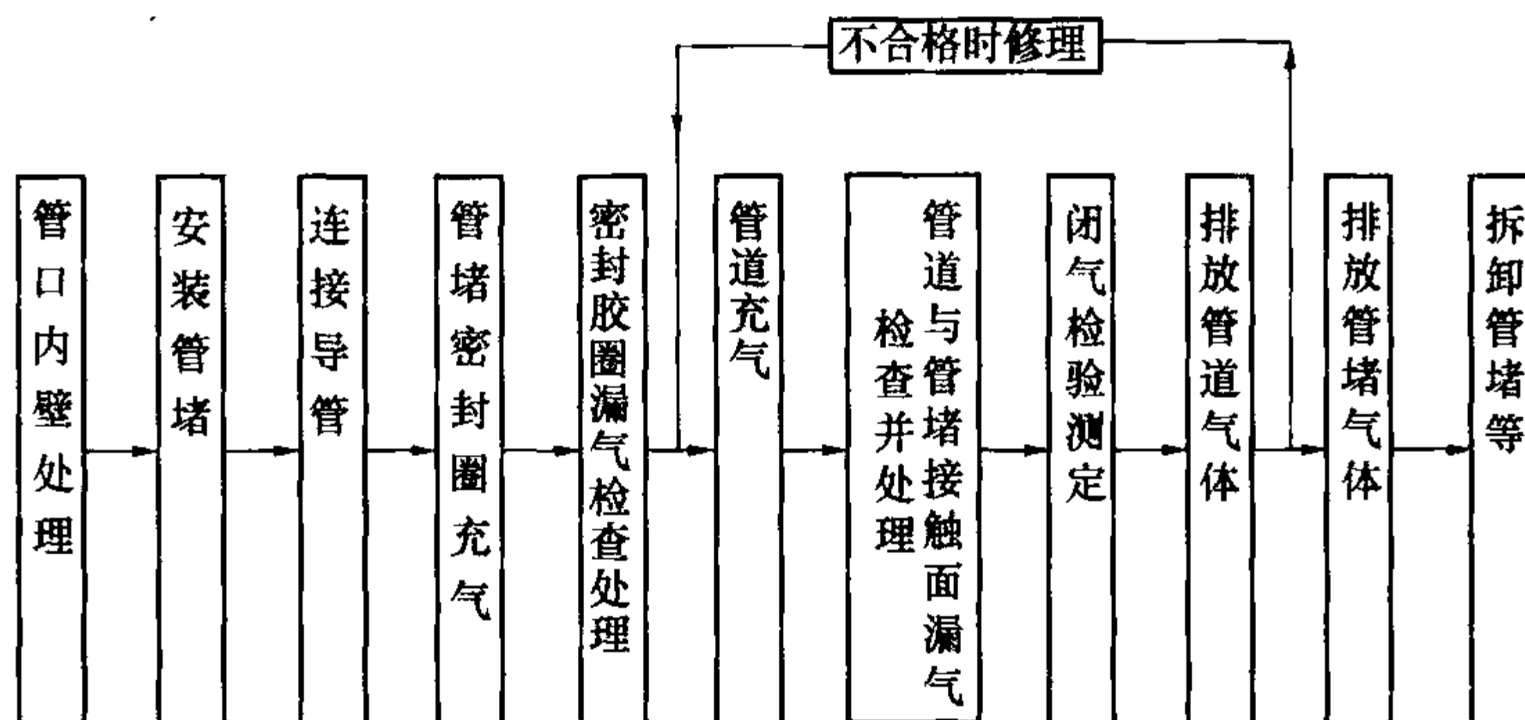
图 E.0.2 管道闭气检验工艺流程图
